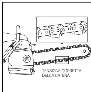
Facile tensionamento della catena
